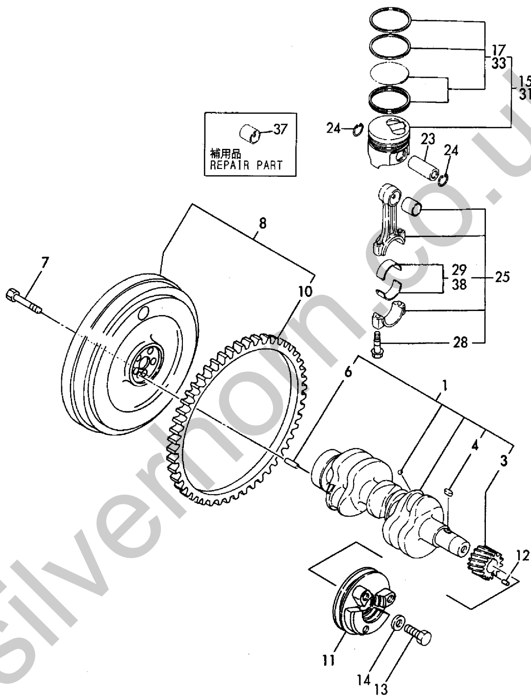
Fig. 7 クランクシャフト&ピストン CRANKSHAFT & PISTON
