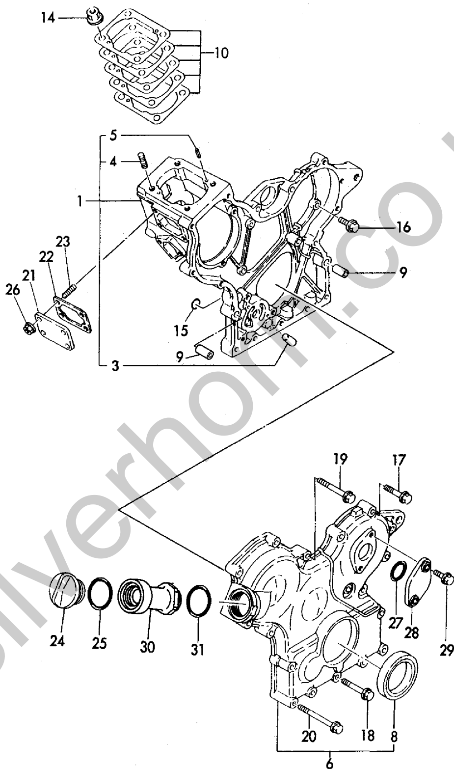
Fig. 2 ギヤケース GEAR HOUSING
