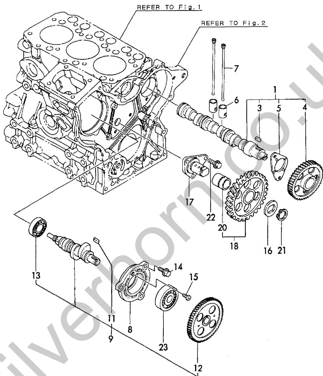
Fig. 6 カムシャフト & 駆動ギヤ CAMSHAFT & DRIVING GEAR
