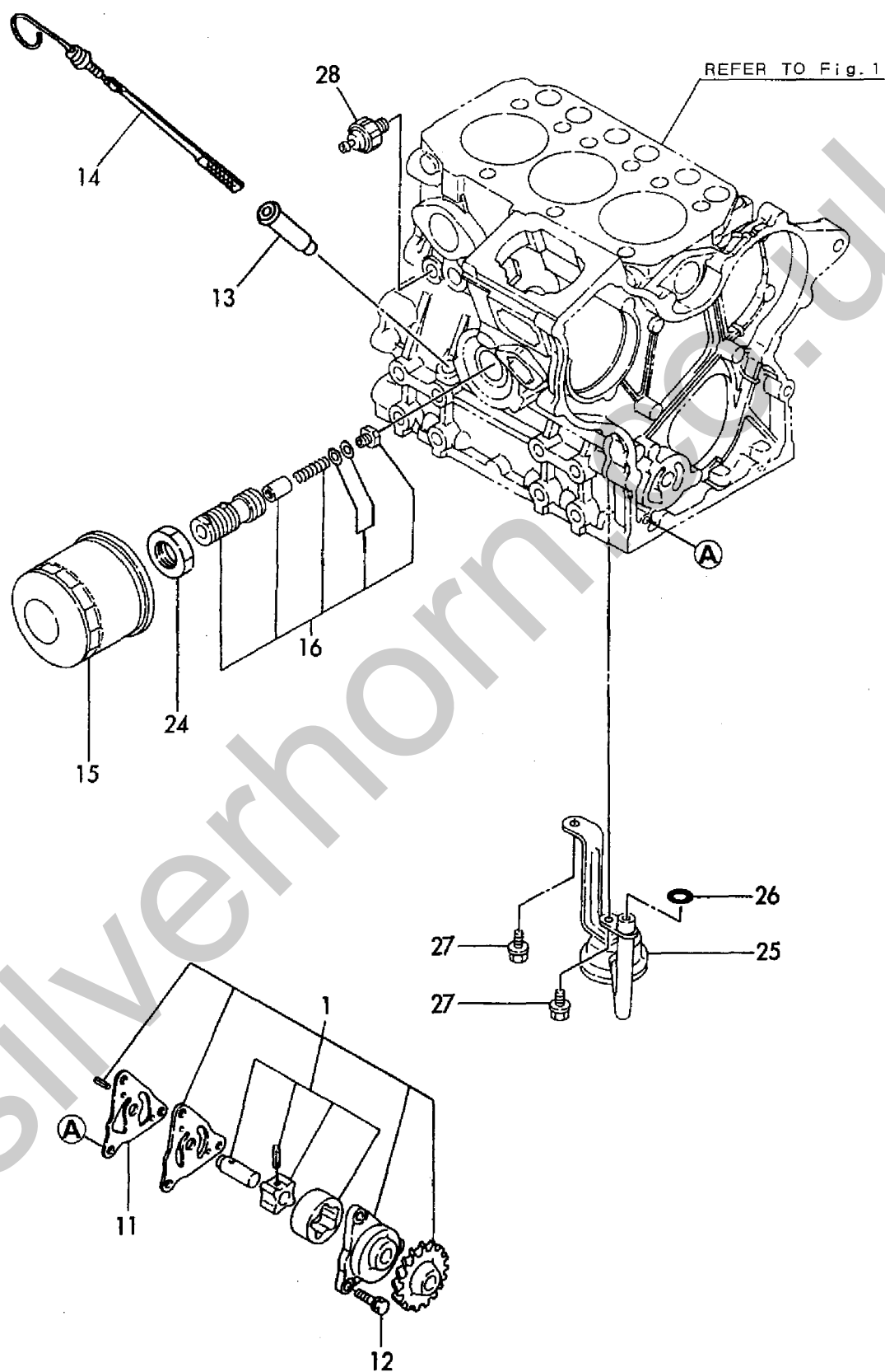
Fig. 8 潤滑油システム LUB. OIL SYSTEM
